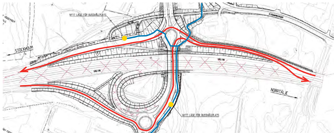
Bild 1: Trafikplats Viggbyholm.
