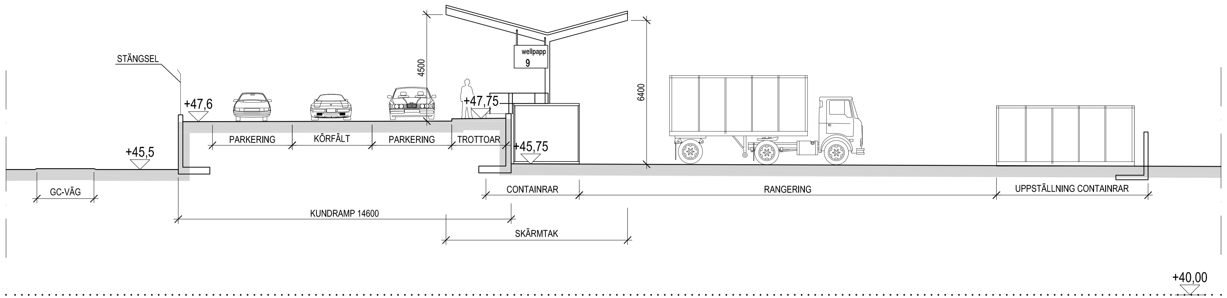
SEKTION A - A
